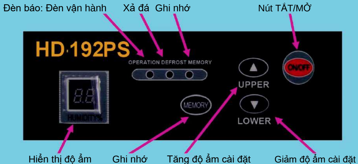
Bảng điều khiển (giống nhau cho cả 3 model)
